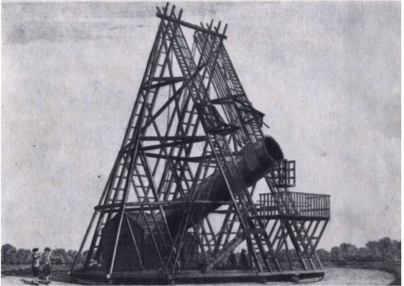
Крупнейший из телескопов Вильяма Гершеля с диаметром зеркала 120 см. сооружение которого завершено в 1789 г.
