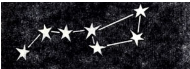
Изменения видимого расположения ярких звезд созвездия Большой Медведицы вследствие их собственных движений: в настоящее время
