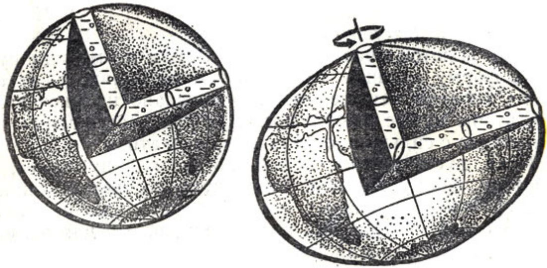
Рассуждение Ньютона о фигуре равновесия вращающейся Земли
