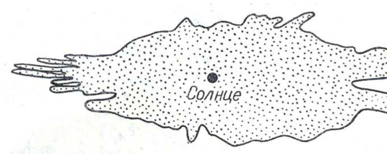
Поперечный разрез Галактики по результатам звездных подсчетов В. Гершеля
