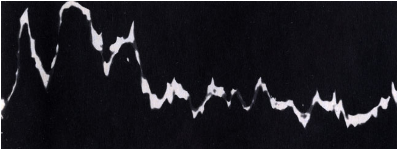
Осциллографическая запись радиоизлучения пульсара. Слева - наблюдаемые пики излучения, справа - уровень 'шума' приемной аппаратуры
