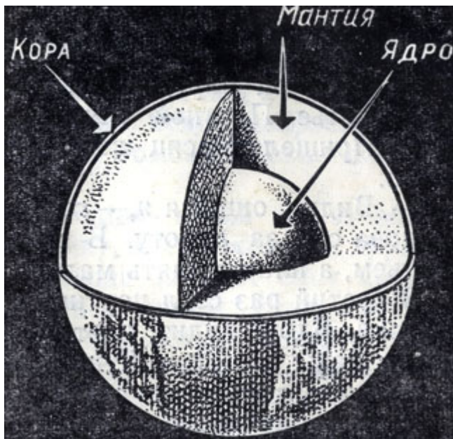
Схематическое изображение внутреннего строения Земли
