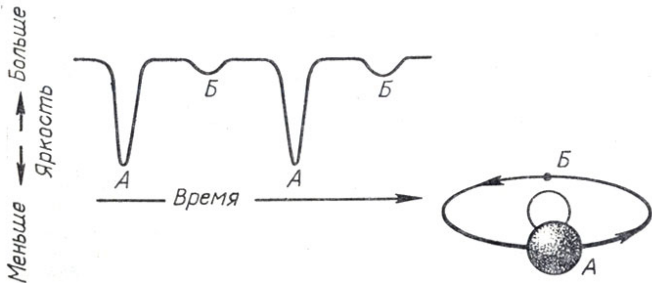
Диаграмма изменения яркости затменно-переменной звезды Алголь
