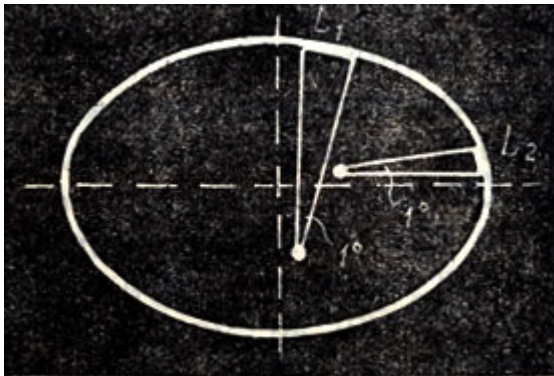
Схема поясняет принцип определения фигуры Земли из измерений двух дуг меридиана в 1^\circ на разных широтах
