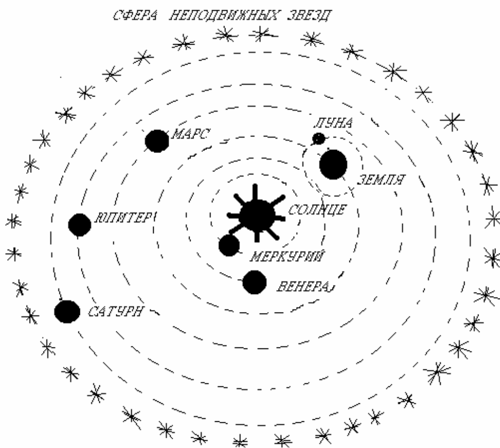
Рис.3. Гелиоцентрическая система Коперника
