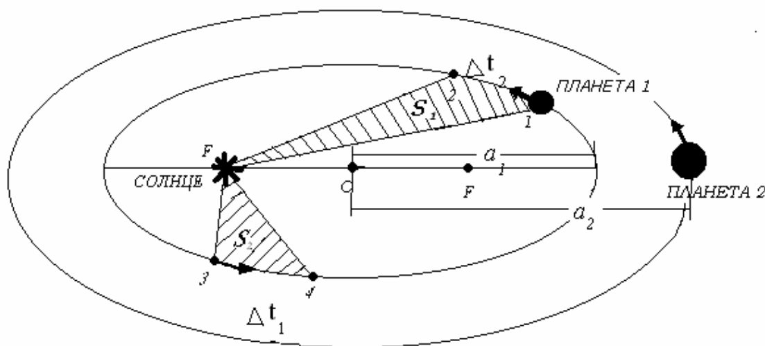
Рис.1. К пояснению законов Кеплера
