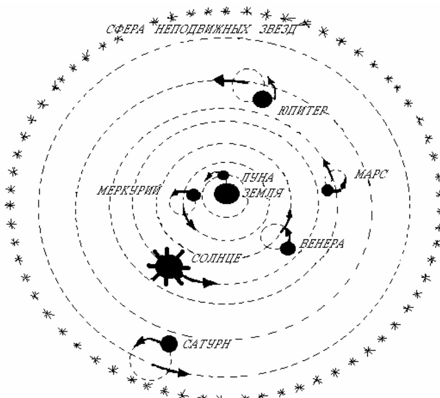
Рис.2. Геоцентрическая система мира
