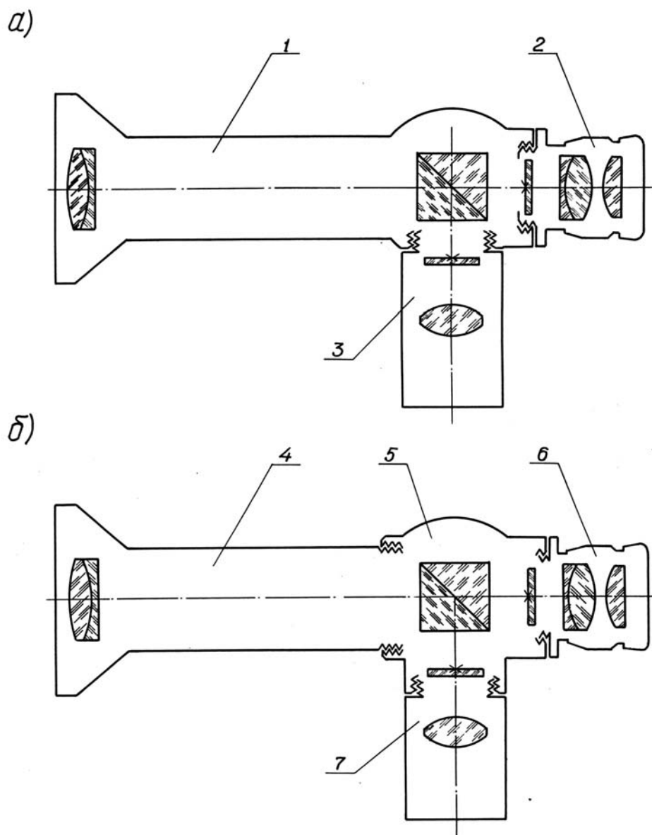
Рис. 9. Два варианта расчленения на узлы конструкции торцовой автоколлимационной трубки
