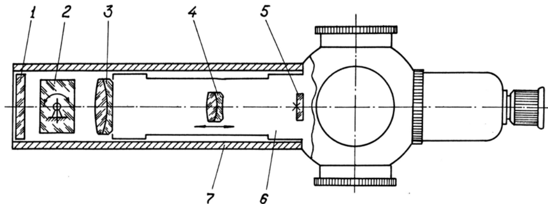
Рис. 17. Конструкция визирной системы трубы ППС-11
