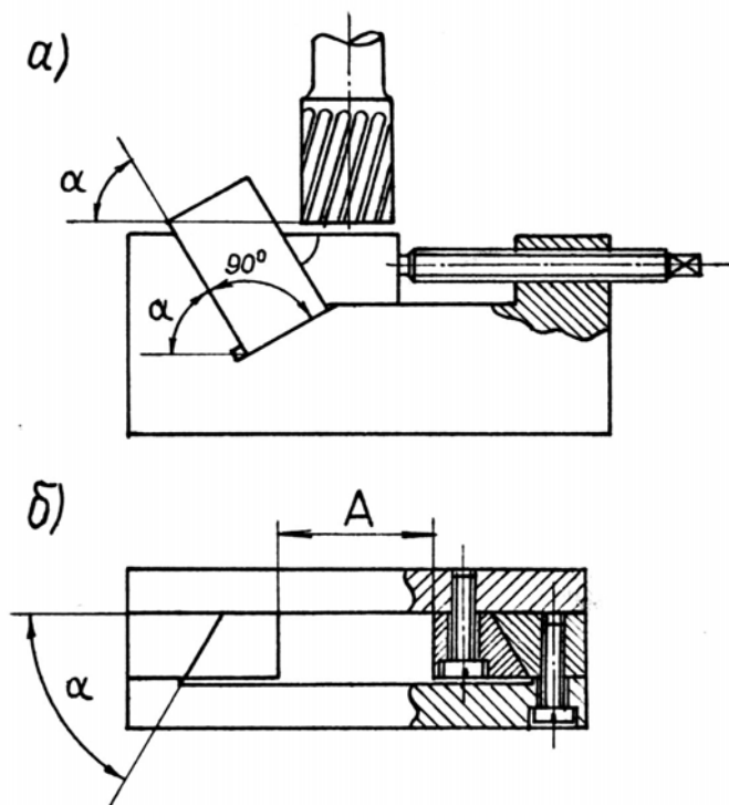
Рис. 22. Изготовление направляющих планок методом «взаимокомпенсирующей технологии» и соответствующая этому методу конструкция направляющих
