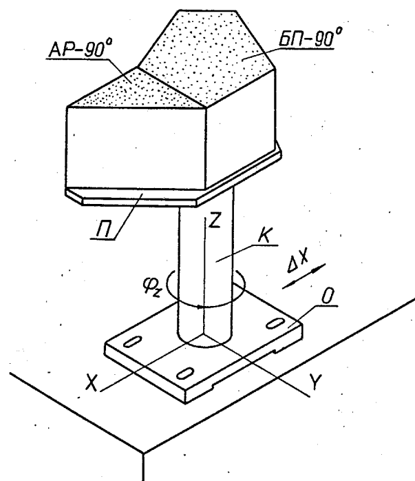
Рис. 29. Технологическая конструкция кронштейна с призмами
