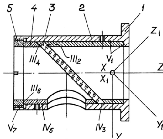
Рис. 20. Крепление в оправе наклонной светоделительной пластины
