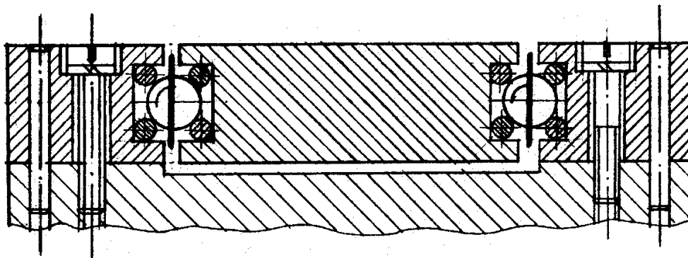
Рис.4. Конструкция проволочных направляющих прямолинейного движения на шариках
