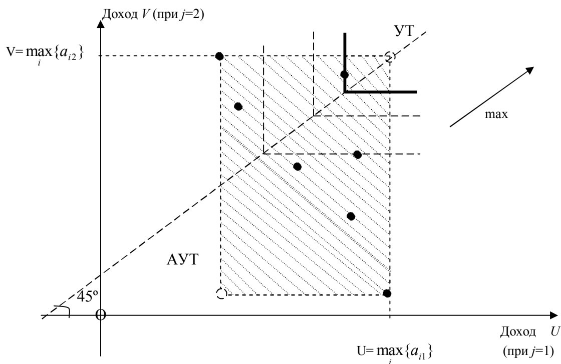
Рис.1.5. Линии уровня MM_{\text{mod}(UT)} -критерия:
