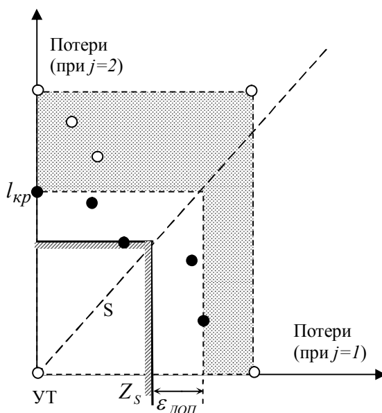
Рис. 3.3. Особенности «преобразования поля потерь» для составных X(S) – критериев при блокировке решений относительно допустимого риска.
