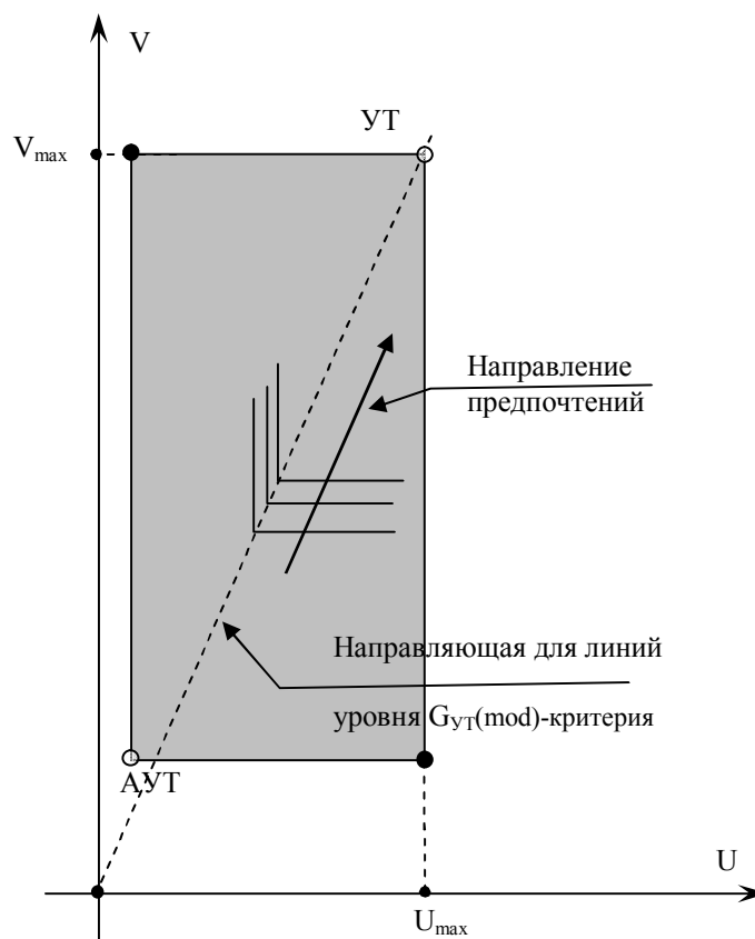
Рис. 4.5. Линии уровня G_{UT}(mod) -критерия.
