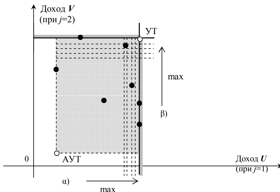
Рис. 2.5б. Специфика выбора для критерия наиболее вероятного исхода.
