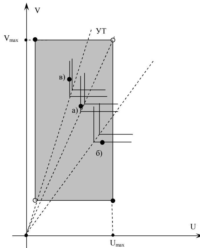
Рис 5.8. Структура линий уровня и особенность оптимального выбора по модифицированному G_{k(UT)}(mod) -критерию: а) при тривиальном простейшем балансе 1:1 для шансов наступления событий \theta_1 и \theta_2 (либо, когда нет необходимости учитывать такой баланс); б) с учетом баланса в пользу события \theta_1 (оси OU); в) с учетом баланса в пользу события \theta_2 (оси OV).
