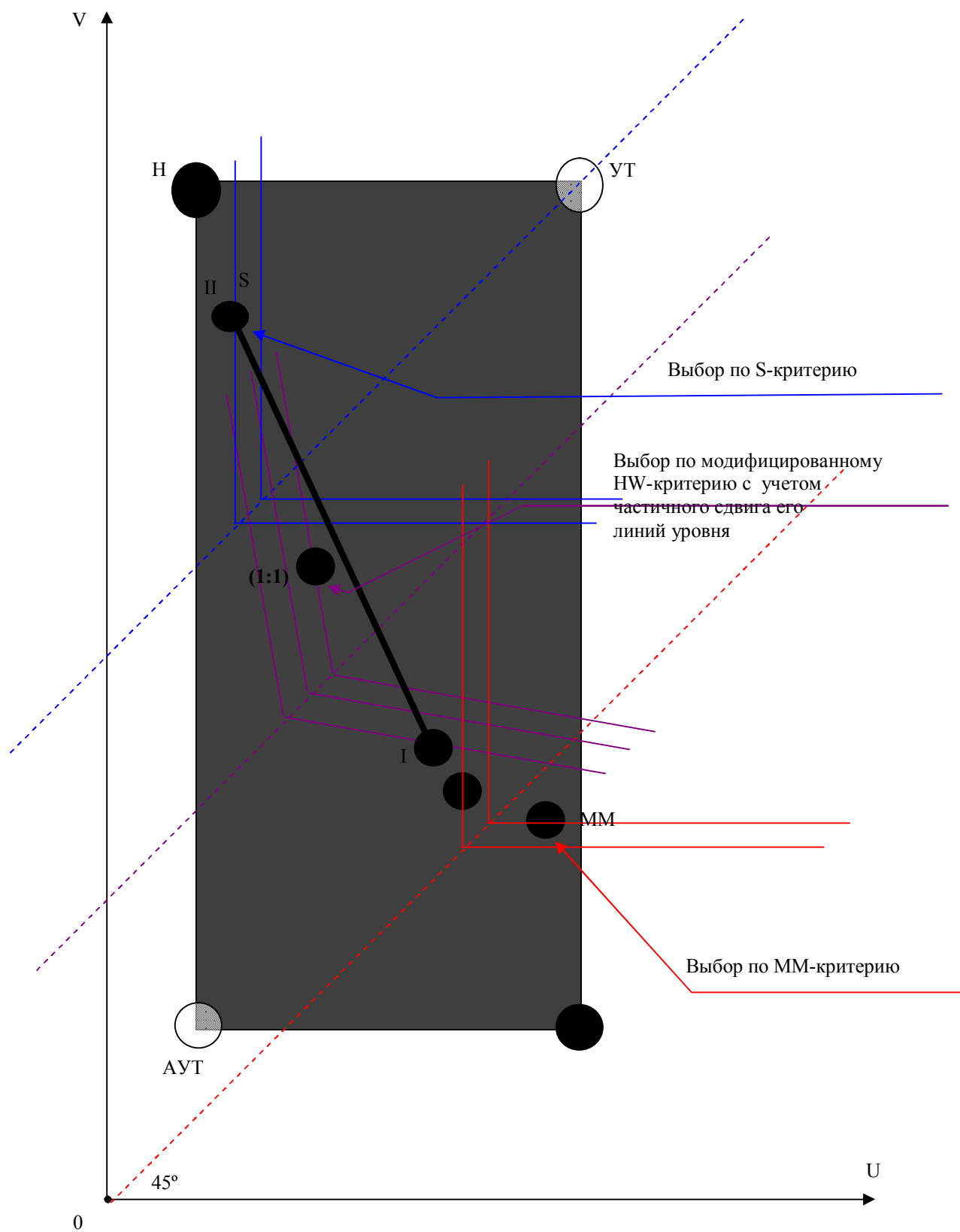
Рис. 5.6b. Выбор в соответствии с модифицированным HW-критерием на основе частичного сдвига линий уровня к утопической точке поля полезностей
