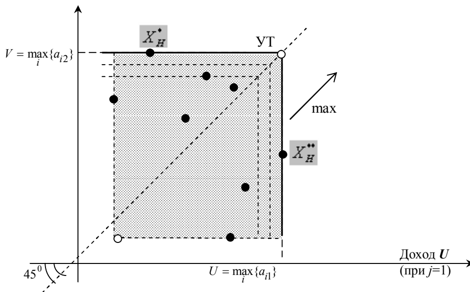
Рис 1.2г. Любое из решений X_H^* и X_H^{**} может быть выбрано в качестве оптимального по H -критерию.
