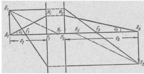
Рис. 5.2. К определению углового увеличения системы. A_1M_1 , A_2M_2 — сопряженные лучи, F_{1,2} — фокусы, H_{1,2} — главные точки, H_1M_1 , H_2M_2 — главные плоскости, N_{1,2} — узлы.
