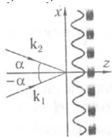
Рис. 6.4. Интерференция плоских волн. Волновые векторы \vec{k}_{1,2} плоских волн лежат в плоскости xz , под углом \pm\alpha к оси z .
