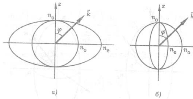
Рис. 12.9. Сфера и эллипсоид показателя преломления для положительного (а) и отрицательного (б) одноосных анизотропных кристаллов
