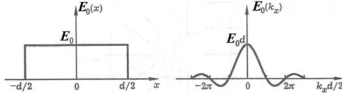
Рис. 9.6. Начальное распределение амплитуды поля E_0(x) и пространственная спектральная амплитуда E_0(k_x) при дифракции плоской монохроматической волны на щели шириной d .
