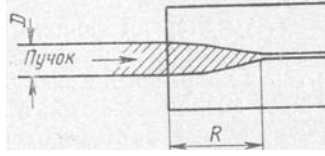
Рис. 15.3. Явление самофокусировки
