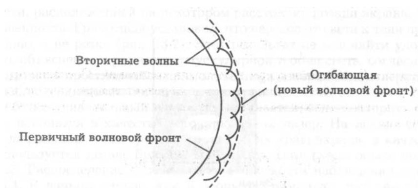
Рис. 8.1. Построение огибающей световой волны по Гюйгенсу
