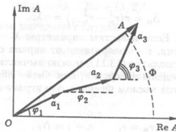
Рис. 8.5. Сложение гармонических колебаний методом векторной диаграммы
