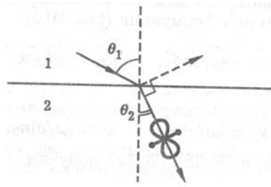
Рис. 11.4. К пояснению эффекта Брюстера
