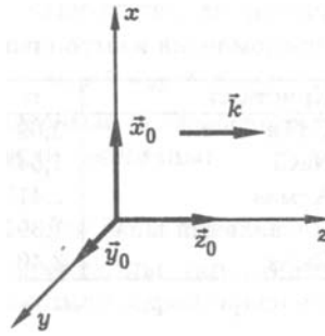
Рис. 12.4. К анализу собственных состояний поляризации световой волны в анизотропном кристалле. Показаны главные оси кристалла x , y , z и волновой вектор световой волны \vec{k}
