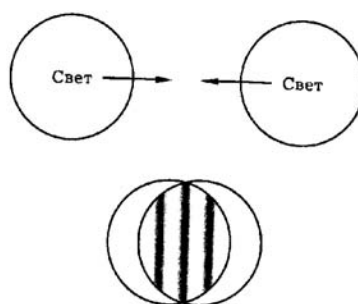
Рис. 6.1. Явление интерференции. При наложение двух световых пучков образуется интерференционная картина — чередование темных и светлых полос, т.е. происходит перераспределение света по пространству: темные полосы соответствуют отсутствию света, светлые — усиленному свету. В пределах темных полос на экране два световых пучка практически полностью гасят друг друга.
