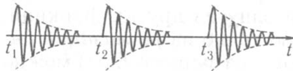
Рис. 2.2. Последовательность цугов, излучаемых атомом какого-либо источника света
