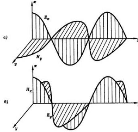
Рис. 1.3. Плоские гармонические волны E_x, H_y (а) и E_y, H_x (б). Здесь показана "мгновенная фотография—распределение полей \vec{E} и \vec{H} как функция координаты z в некоторый момент времени t для волн, бегущих слева направо.
