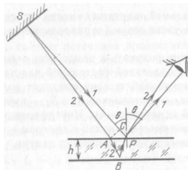
Рис. 6.8. Схема наблюдения полос равной толщины.
