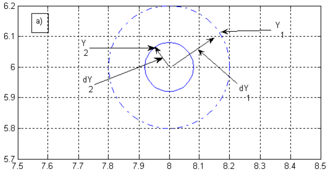
Рис. 5а. Погрешности \delta y_1 и \delta y_2 коллинеарны собственным векторам матрицы A_t^T A_t .
