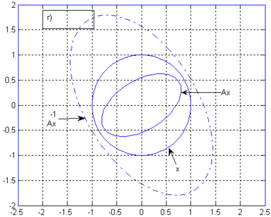
Рис. 6г. Отображение окружности матрицей четвертого типа: 0 < \sigma_{\min} < \sigma_{\max} < 1 , \text{cond}(\mathbf{A}) = 1.78 .
