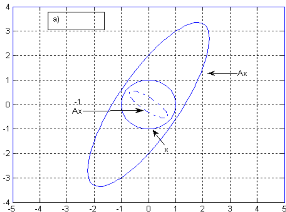
Рис. 6а. Отображение окружности матрицей первого типа: \sigma_{\min} > 1 , \text{cond}(\mathbf{A}) = 3.3 .
