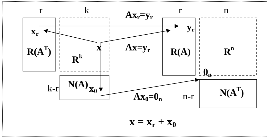
Рис. 1. Условное изображение расщепления пространств \mathbb{R}^k и \mathbb{R}^n .
